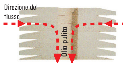
Corpo della cartuccia (Sezione trasversale) - L'olio scorre nella cartuccia filtrante di profondità CJC™ radialmente dall'esterno verso l'interno.
